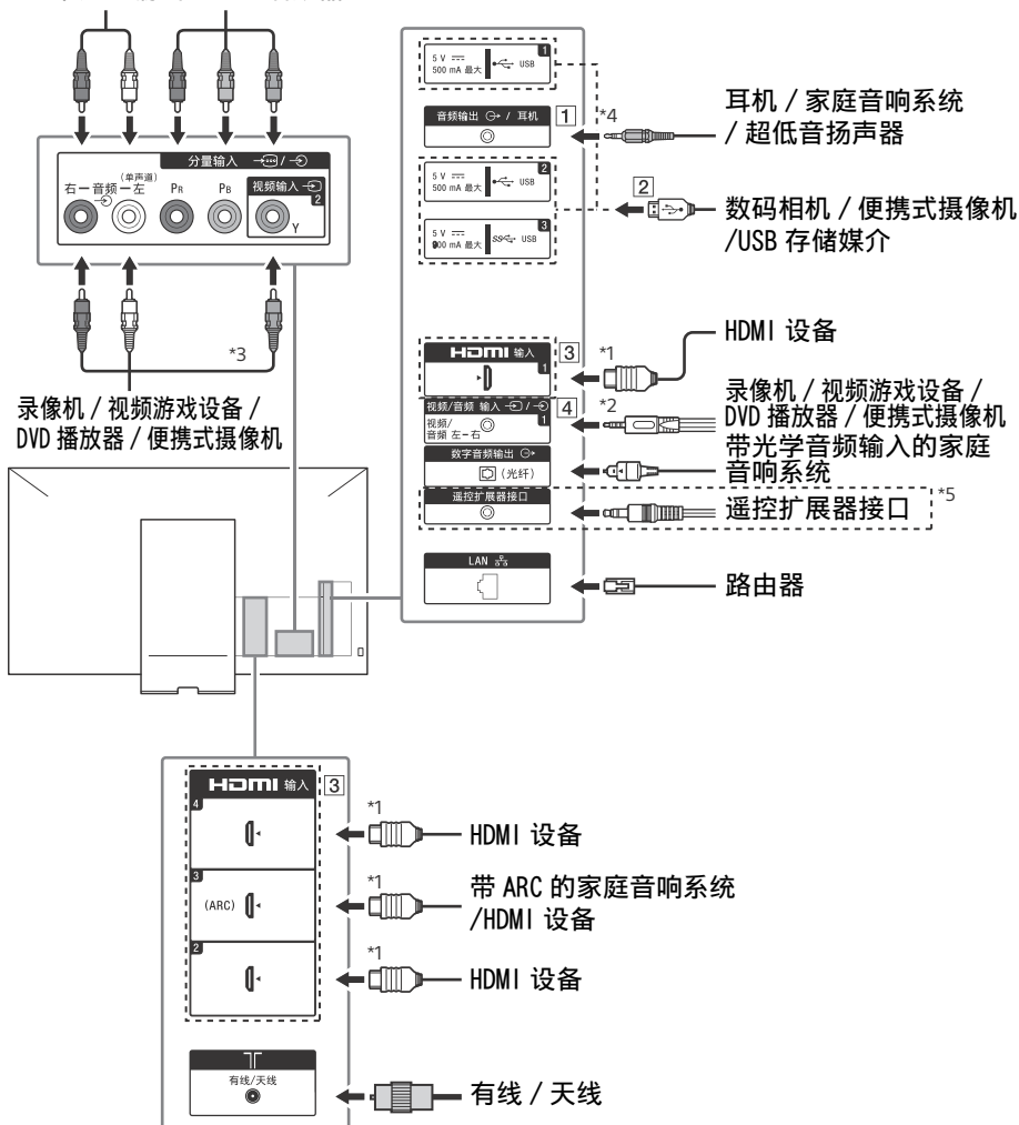
带分量输出的 DVD 播放器
