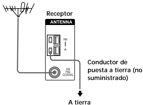
Antena exterior de FM
